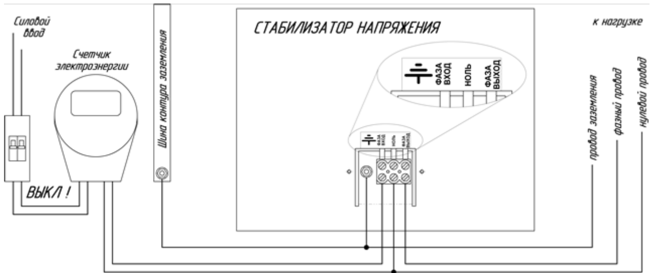
Рисунок 1. Рекомендуемая схема подключения стабилизатора к сети.
